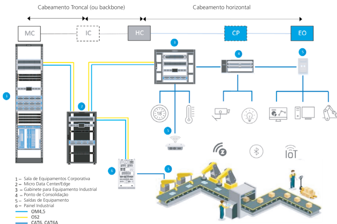
Figura 2 Topologia típica de uma rede Industrial
